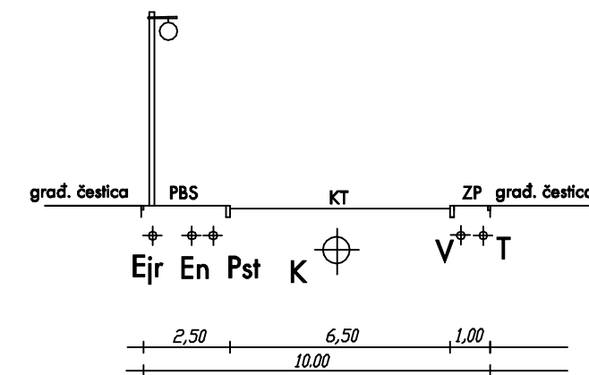
UK - presjek 1-1
