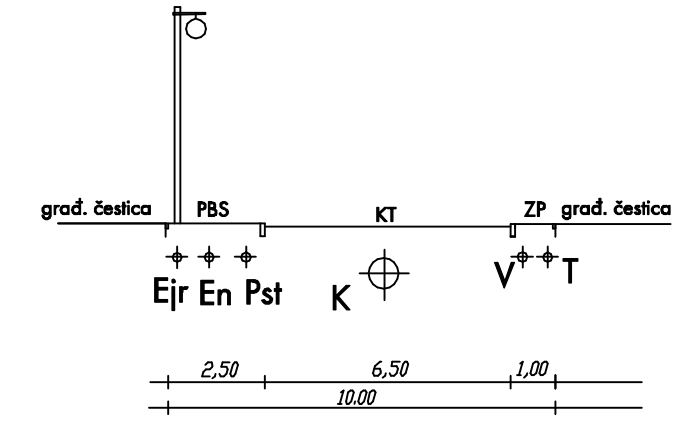
UK - presjek 1-1
