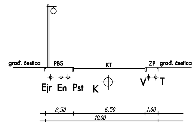
UK - presjek 1-1
